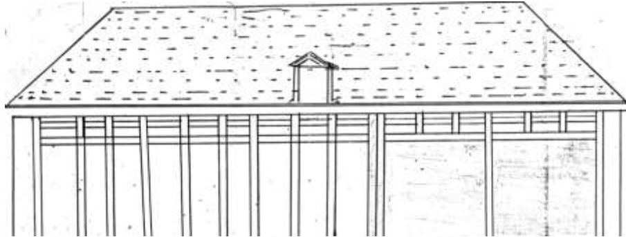
A tetőszerkezet sémája kiugró tetőablakkal a mai Hajdúkerület utca felől. 1814.
